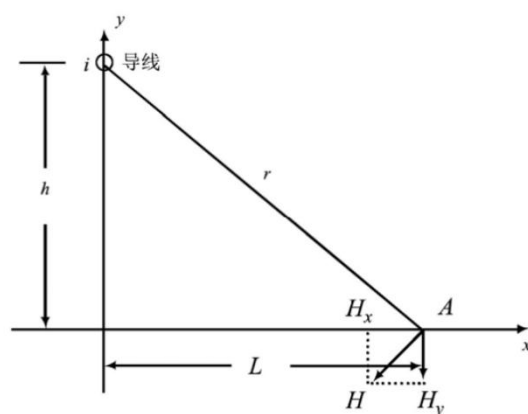
图 3 磁场向量图
