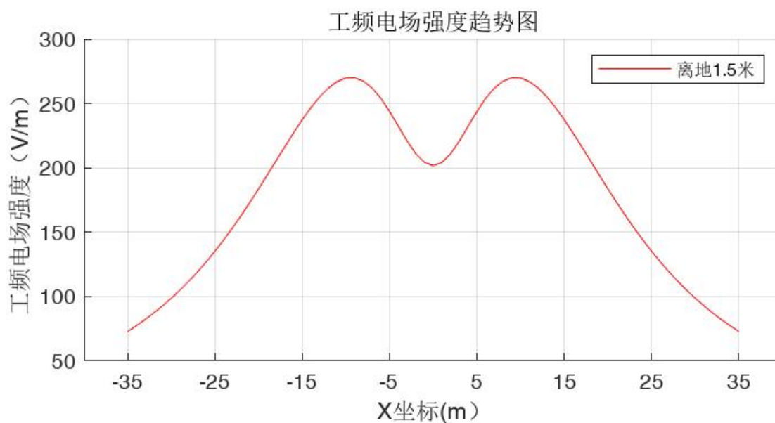
图 4-1 单回 110-DA31D-DJC1 塔型地面 1.5m 处工频电场强度趋势示意图
