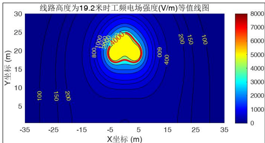
图 4-3 单回 110-DA31D-DJC1 塔型线高 19.2m 时工频电场强度预测结果等值线图
