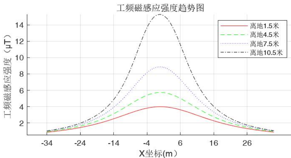
图 4-6 110GJ90 塔型地面 1.5m、4.5m、7.5m、10.5m 处处工频磁感应强度趋势示意图
