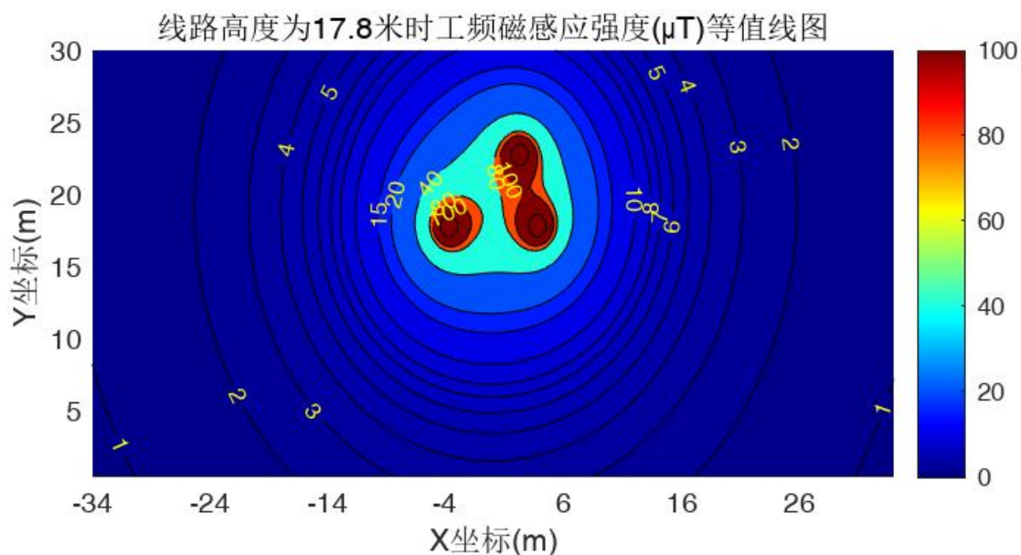
图 4-8 110GJ90 塔型线高 17.8m 时工频磁感应强度预测结果等值线图
