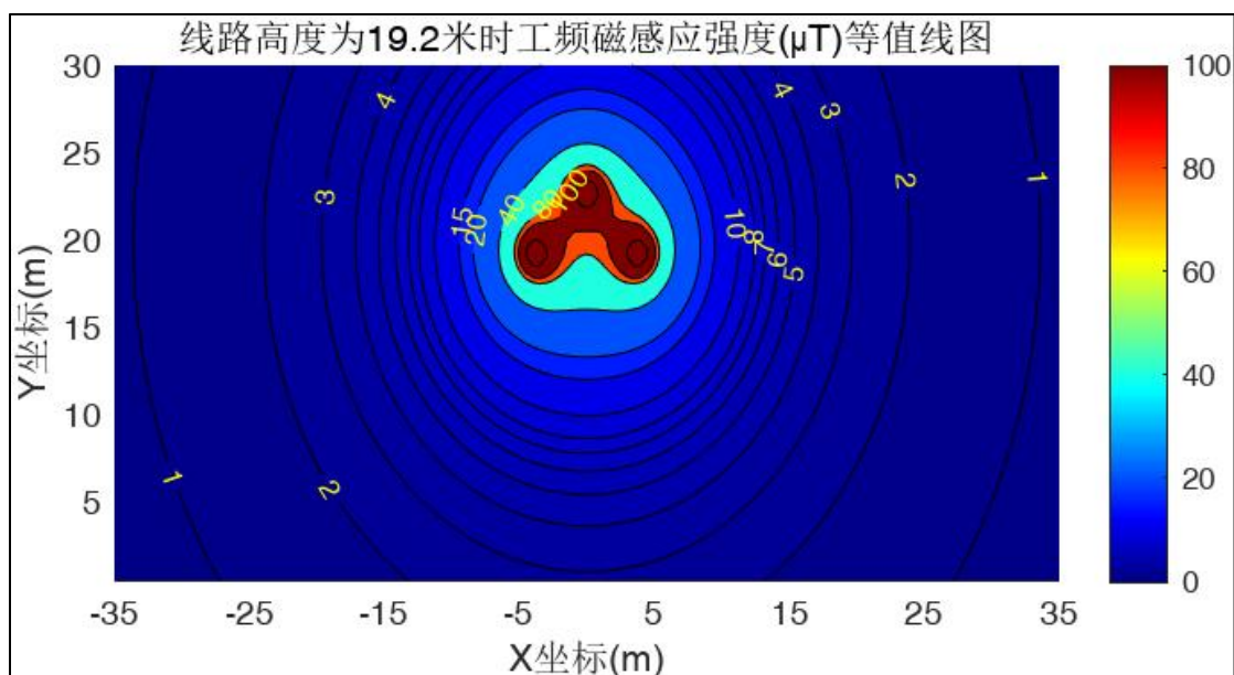
图 4-4 单回 110-DA31D-DJC1 型线高 19.2m 时工频磁感应强度预测结果等值线图
