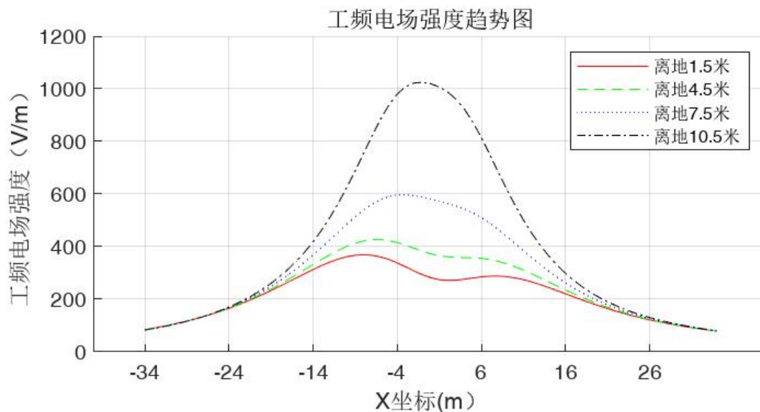
图 4-5 110GJ90 塔型地面 1.5m、4.5m、7.5m、10.5m 处工频电场强度趋势示意图
