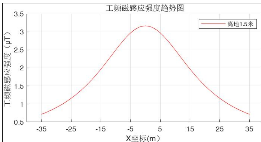
图 4-2 单回 110-DA31D-DJC1 塔型地面 1.5m 处工频磁感应强度趋势示意图
