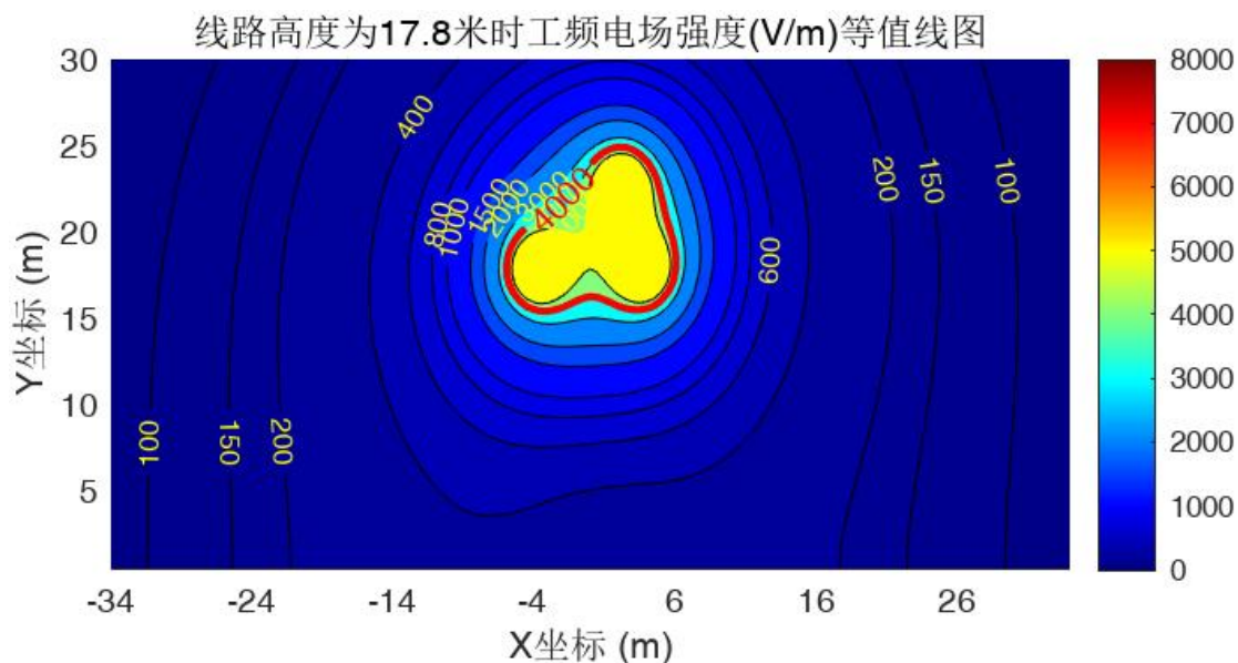
图 4-7 110GJ90 塔型线高 17.8m 时工频电场强度预测结果等值线图
