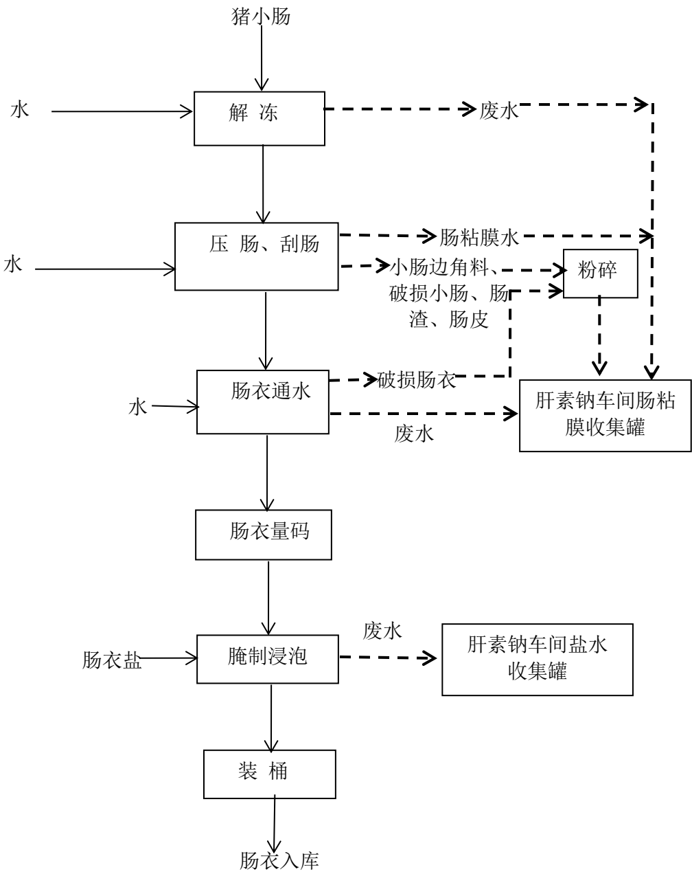
图2.2-1 肠衣工艺流程及产污环节图
