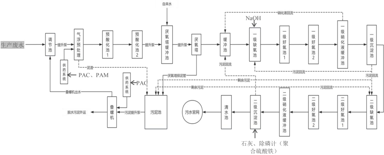
图5.2-1 本项目废水处理措施工艺流程
