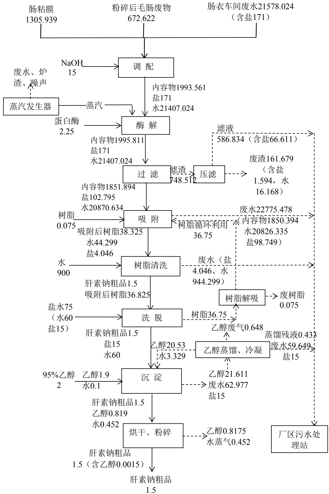
图 2.2-4 肝素钠物料平衡图 单位: t/a
