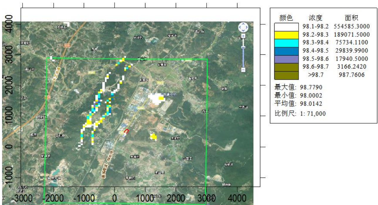
图4.1-22 PM10 95%保证率日平均浓度分布图（单位： \mu\text{g}/\text{m}^3 ）
