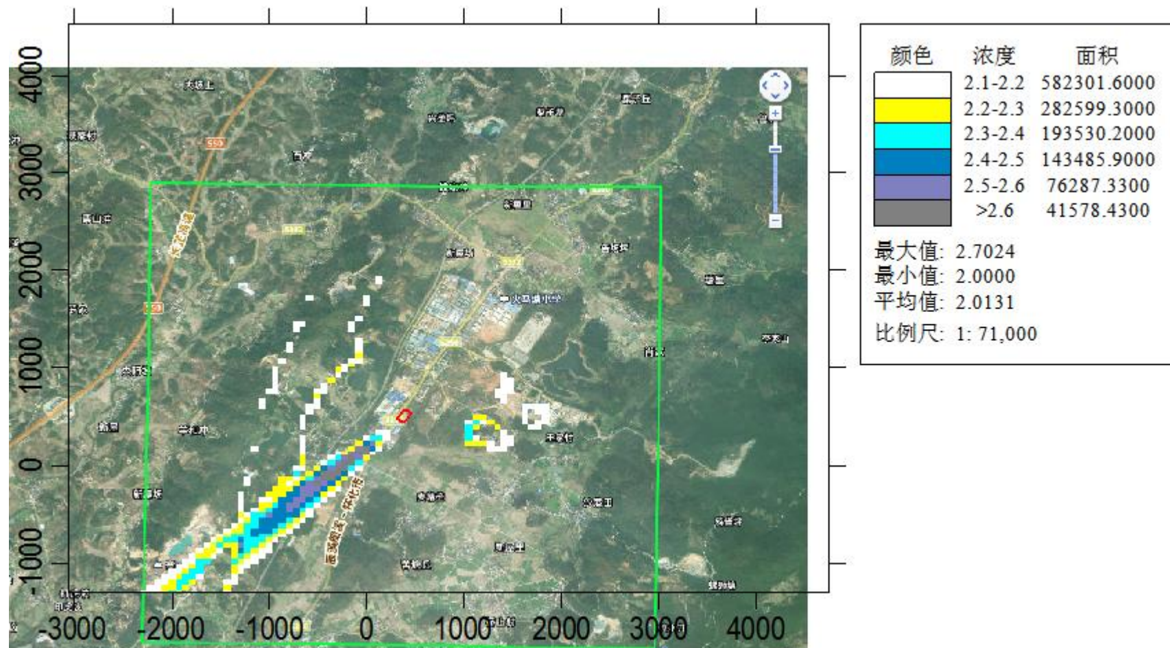
图4.1-25 叠加后硫化氢小时平均浓度分布图 (单位: \mu\text{g}/\text{m}^3 )
