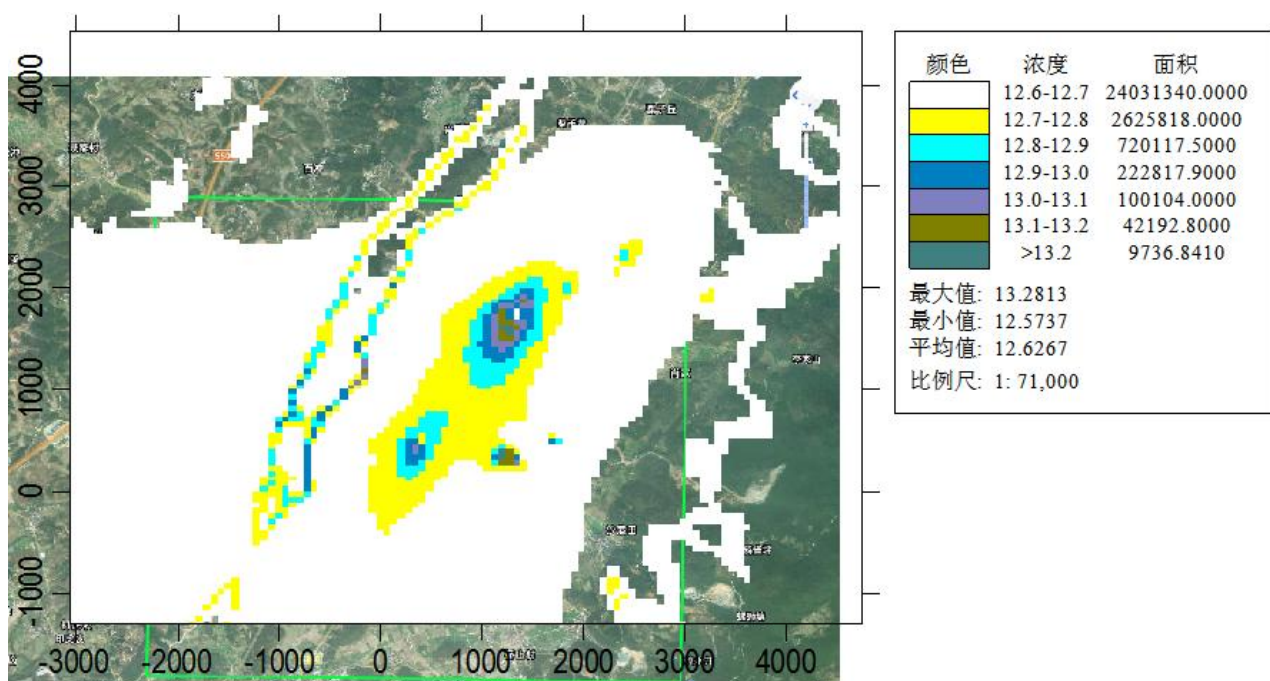
图4.1-21 叠加后NO 2 年平均浓度分布图 (单位: \mu\text{g}/\text{m}^3 )
