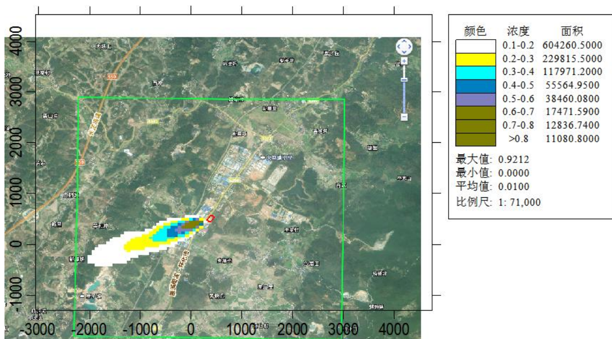
图 4.1-7 SO 2 最大小时平均浓度分布图 (单位: ug/m 3 )
