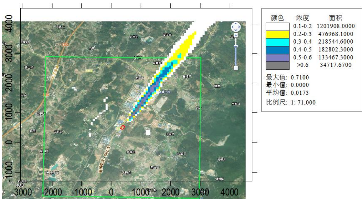
图 4.1-16 硫化氢最大小时平均浓度分布图 (单位: \mu\text{g}/\text{m}^3 )
