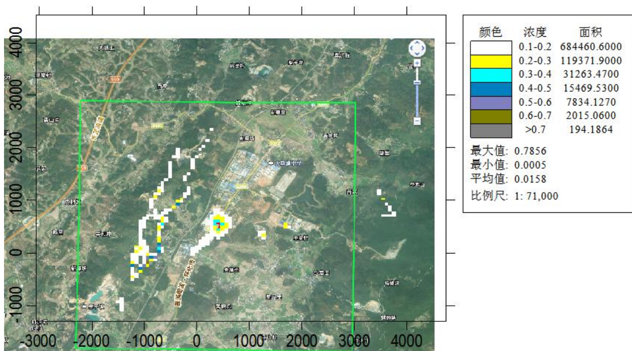
图4.1-11 NO 2 最大日平均浓度分布图（单位: ug/m 3 ）
