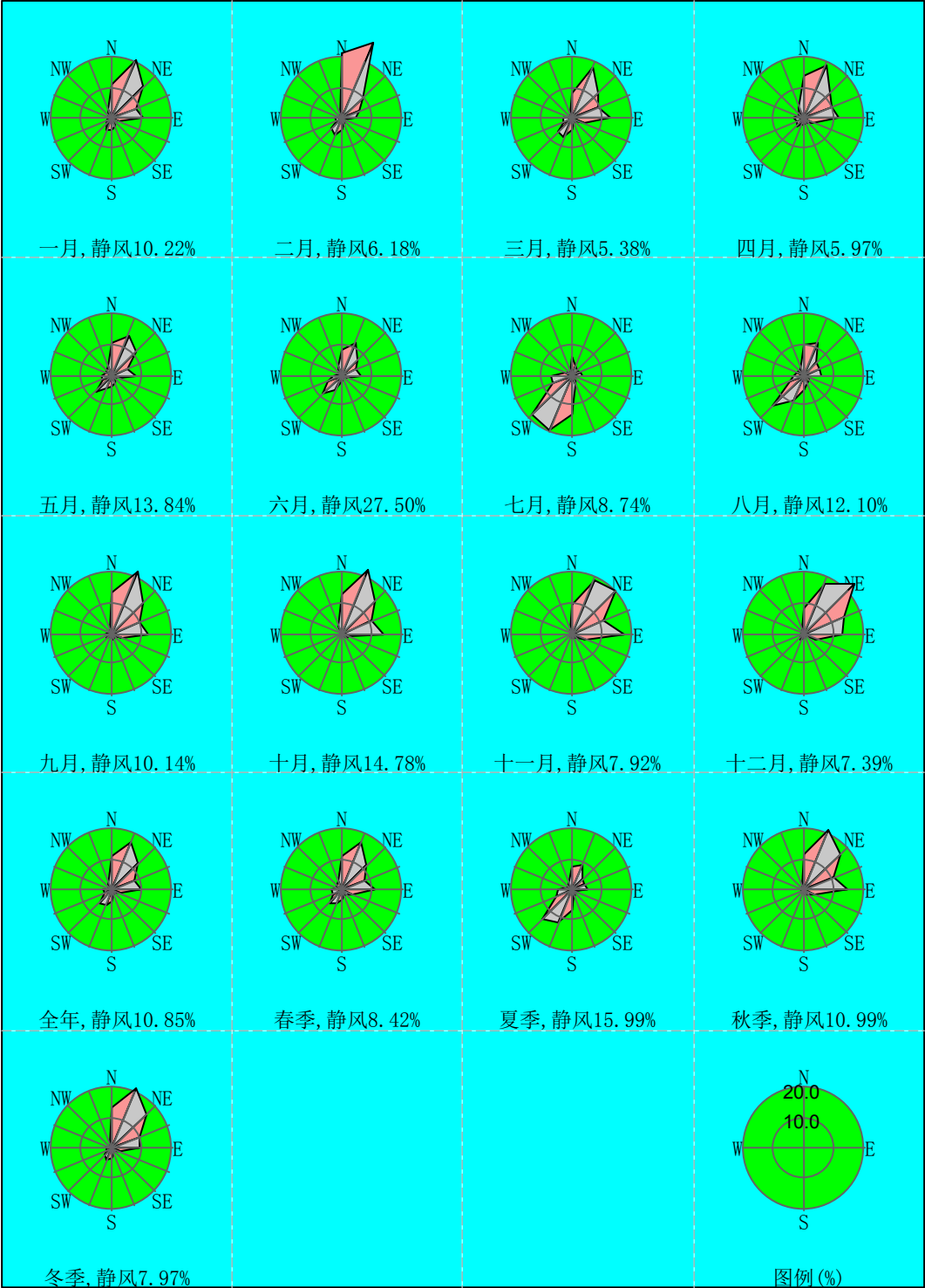
图 4.1-5 怀化市 2024 年风频玫瑰图
