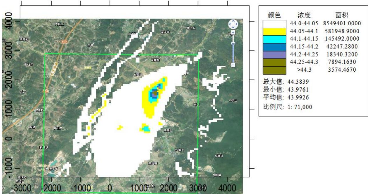
图4.1-22 PM10 95%保证率日平均浓度分布图（单位： \mu\text{g}/\text{m}^3 ）
