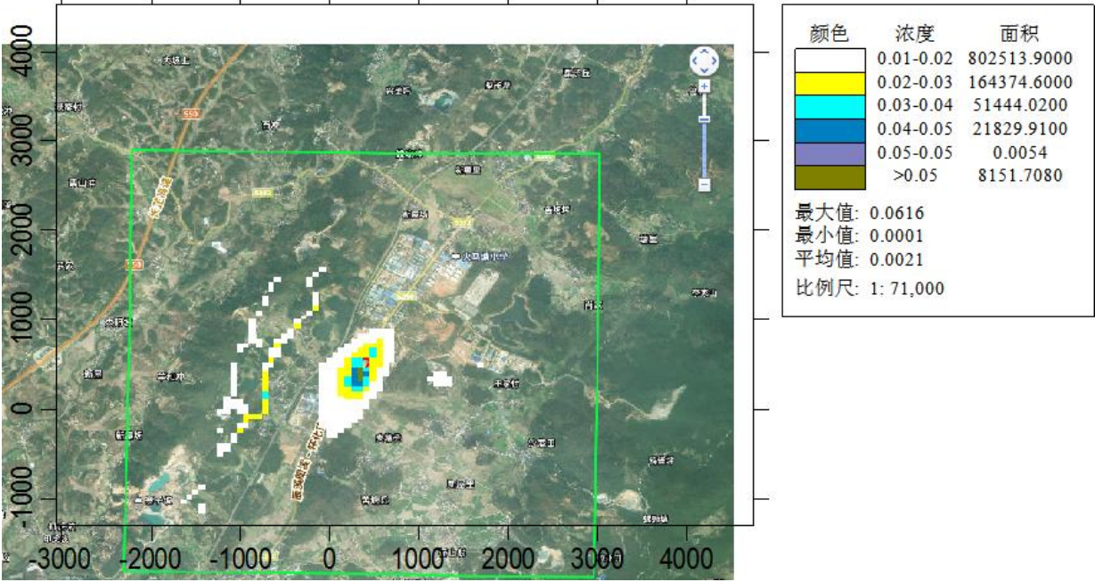
图 4.1-14 PM 10 最大年平均浓度分布图 (单位: ug/m 3 )
