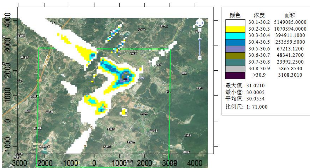
图4.1-20 NO 2 98%保证率日平均浓度分布图 (单位: \mu\text{g}/\text{m}^3 )
