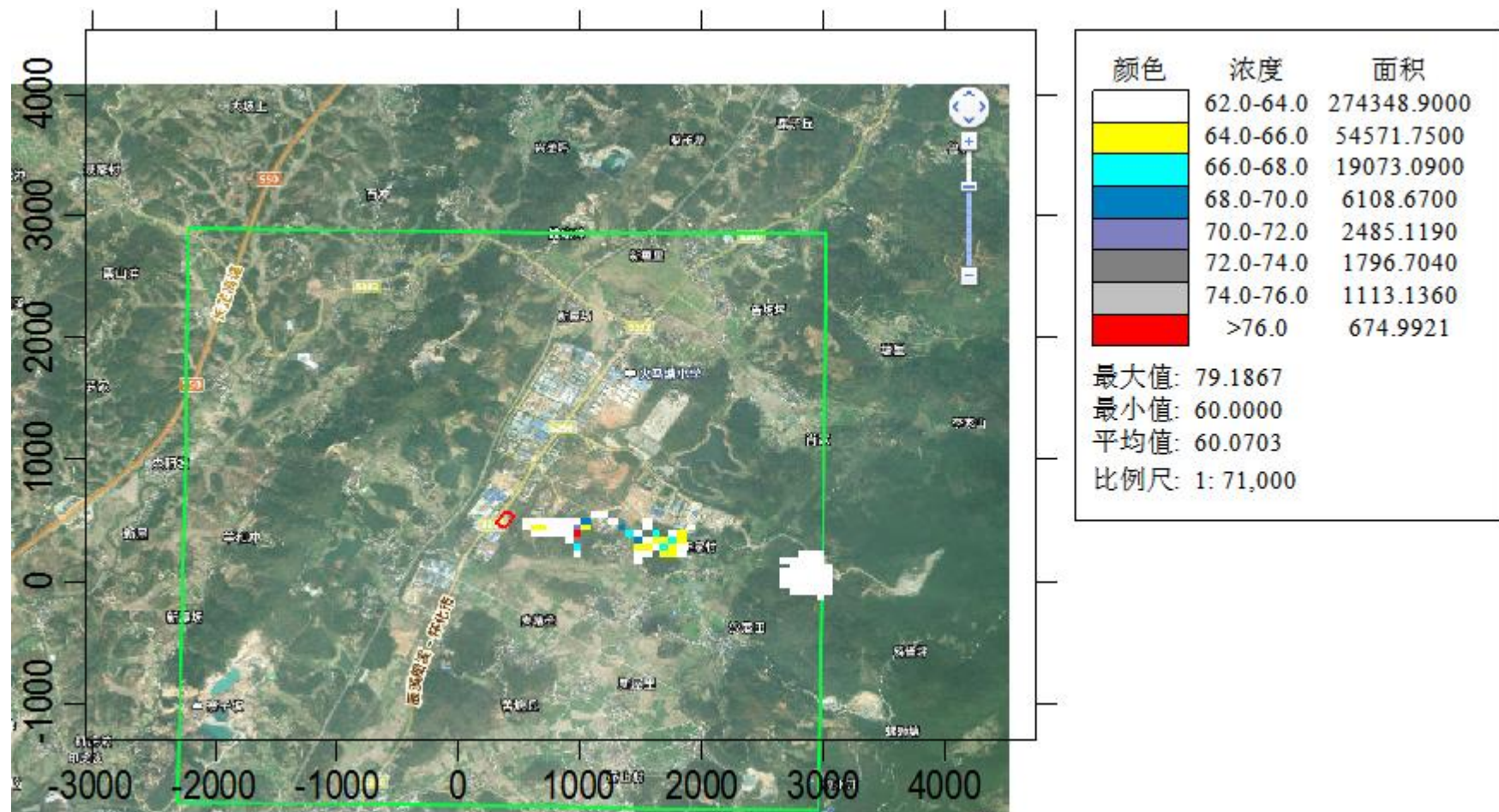
图4.1-24 叠加后氨气小时平均浓度分布图（单位： \mu\text{g}/\text{m}^3 ）
