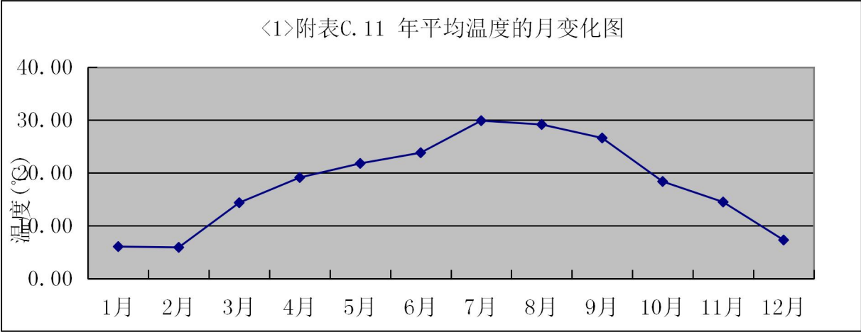
图 4.1-2 怀化市 2024 年平均温度月变化图
