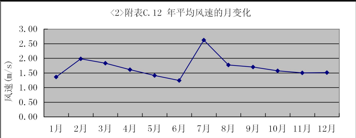
图 4.1-3 怀化市 2024 年平均风速月变化图
