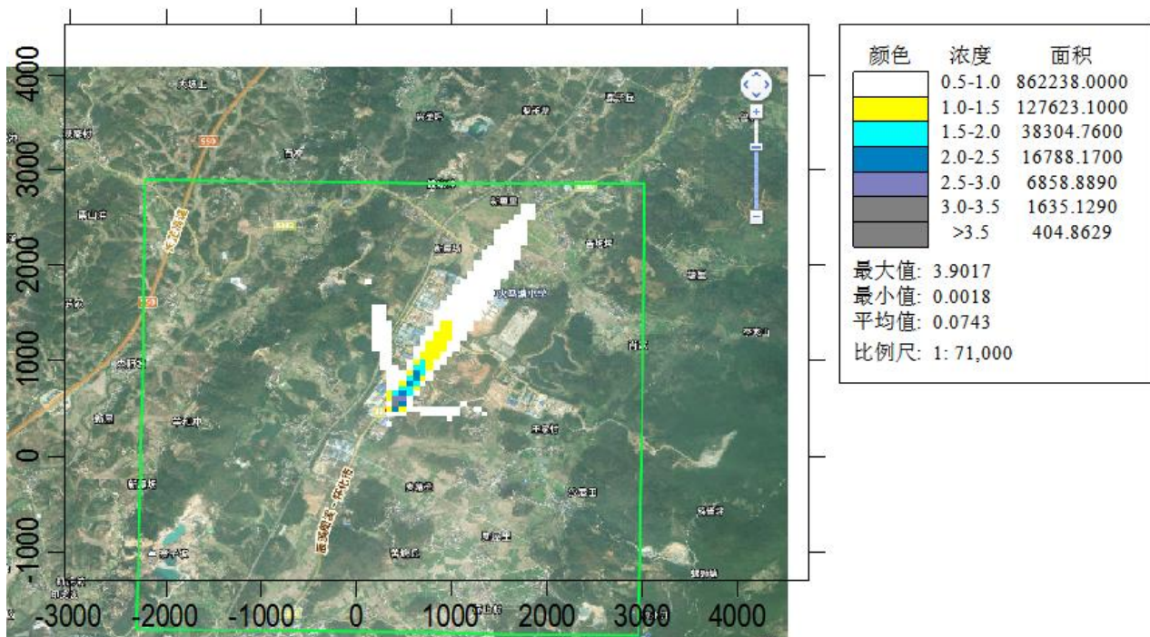
图 4.1-17 TVOC 最大 8 小时平均浓度分布图 (单位: \mu\text{g}/\text{m}^3 )
