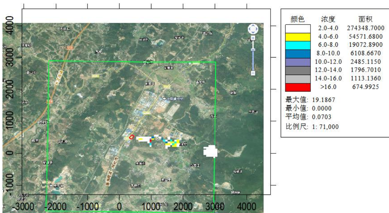
图 4.1-15 氨气最大小时平均浓度分布图 (单位: \mu\text{g}/\text{m}^3 )
