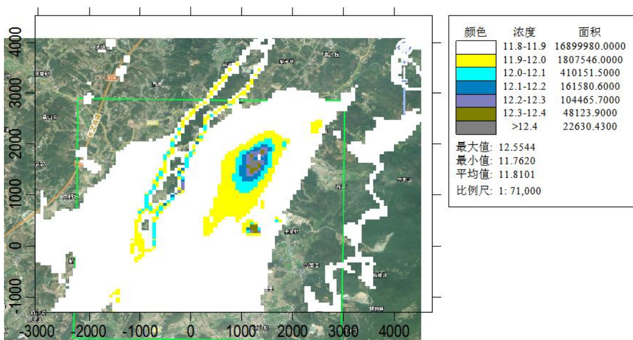
图4.1-19 叠加后SO 2 年平均浓度分布图（单位：ug/m 3 ）
