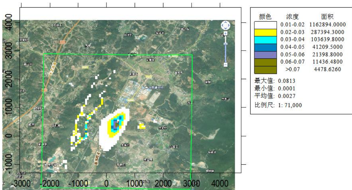
图 4.1-9 SO 2 最大年平均浓度分布图（单位：ug/m 3 ）
