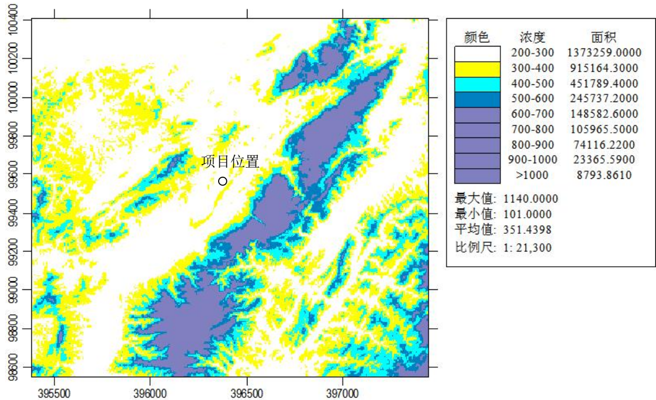
图 4.1-6 项目所在区域地形等值线示意图
