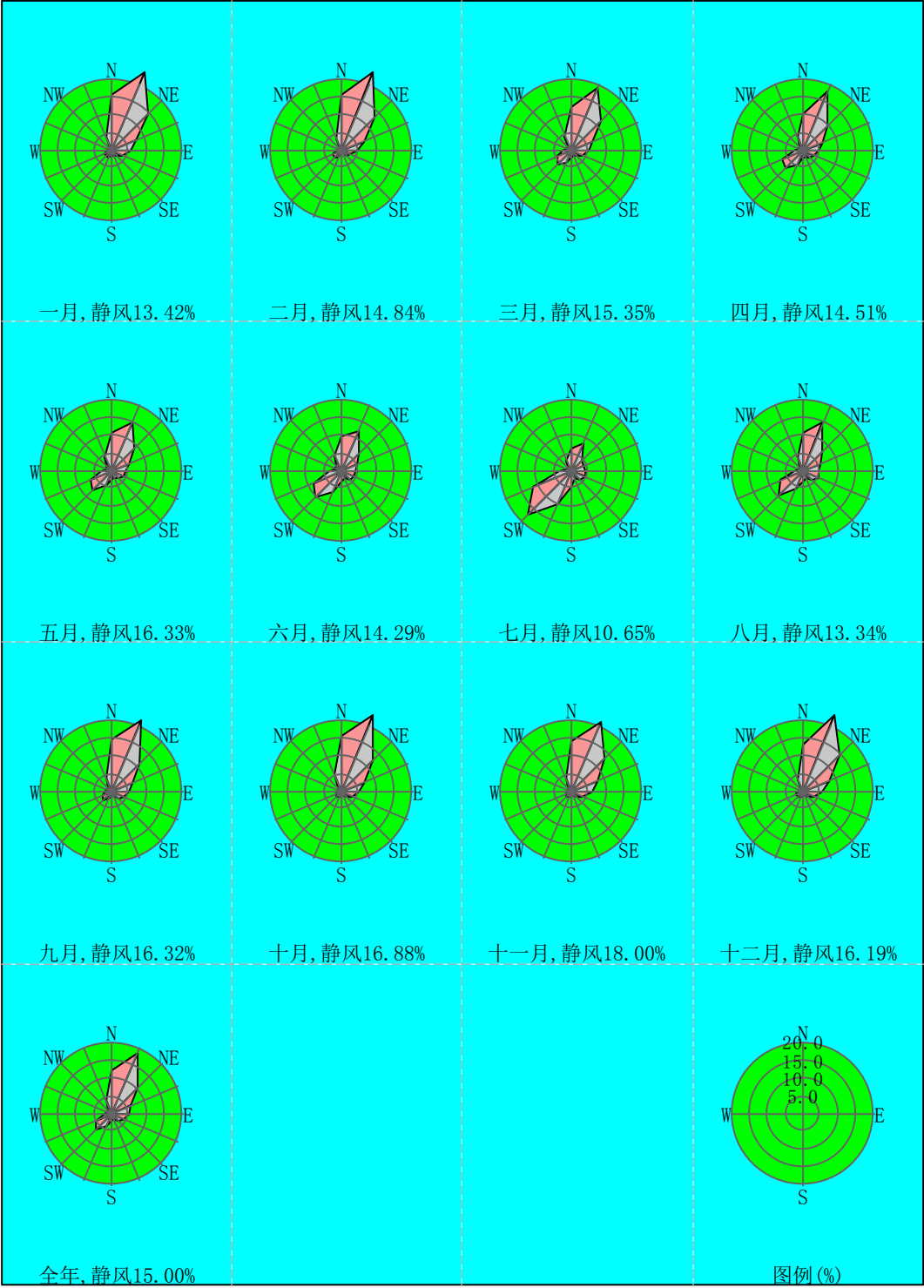
图4.1-1 怀化市近20年月平均风频风玫瑰图
