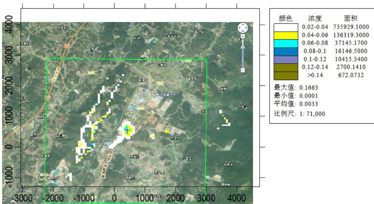
图4.1-8 SO 2 最大日平均浓度分布图 (单位: ug/m 3 )
