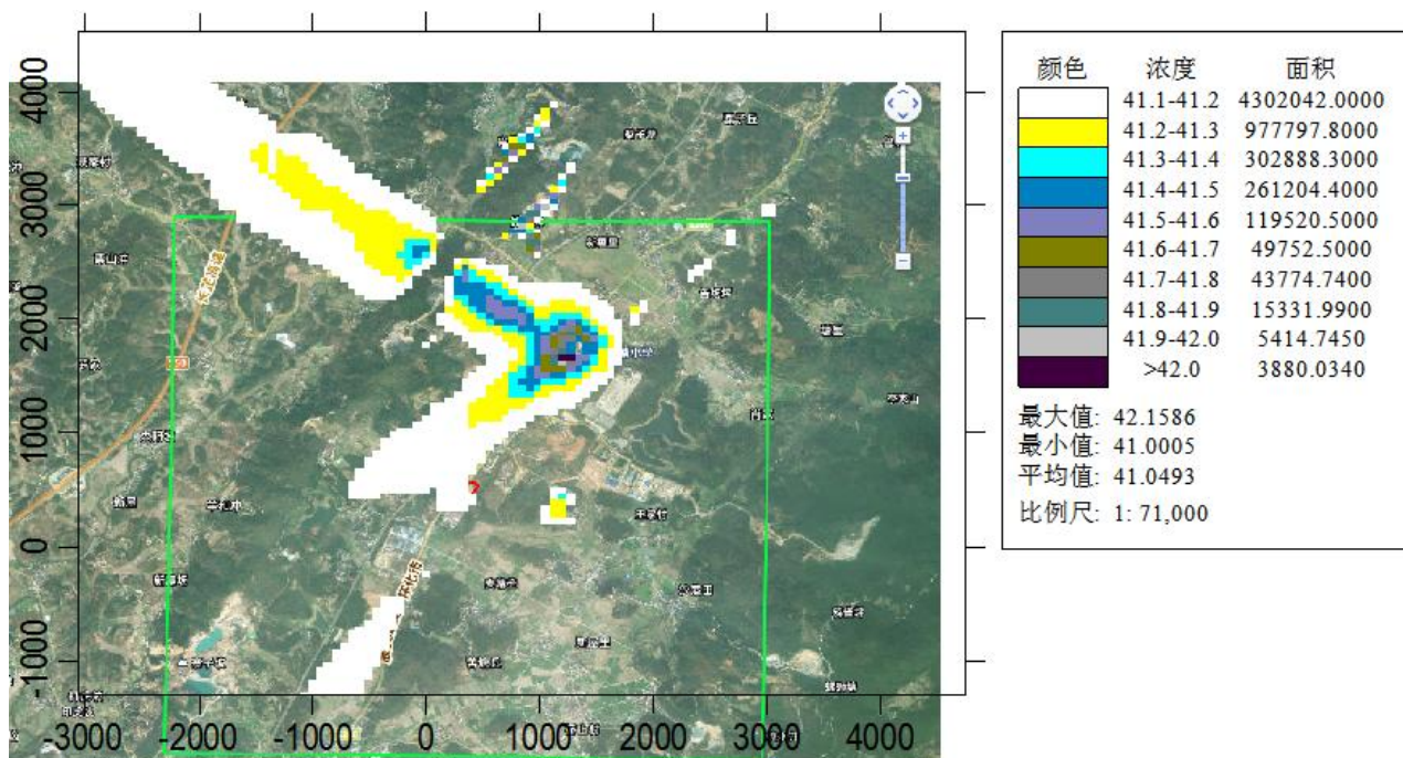
图 4.1-18 SO 2 98%保证率日平均浓度分布图（单位：ug/m 3 ）
