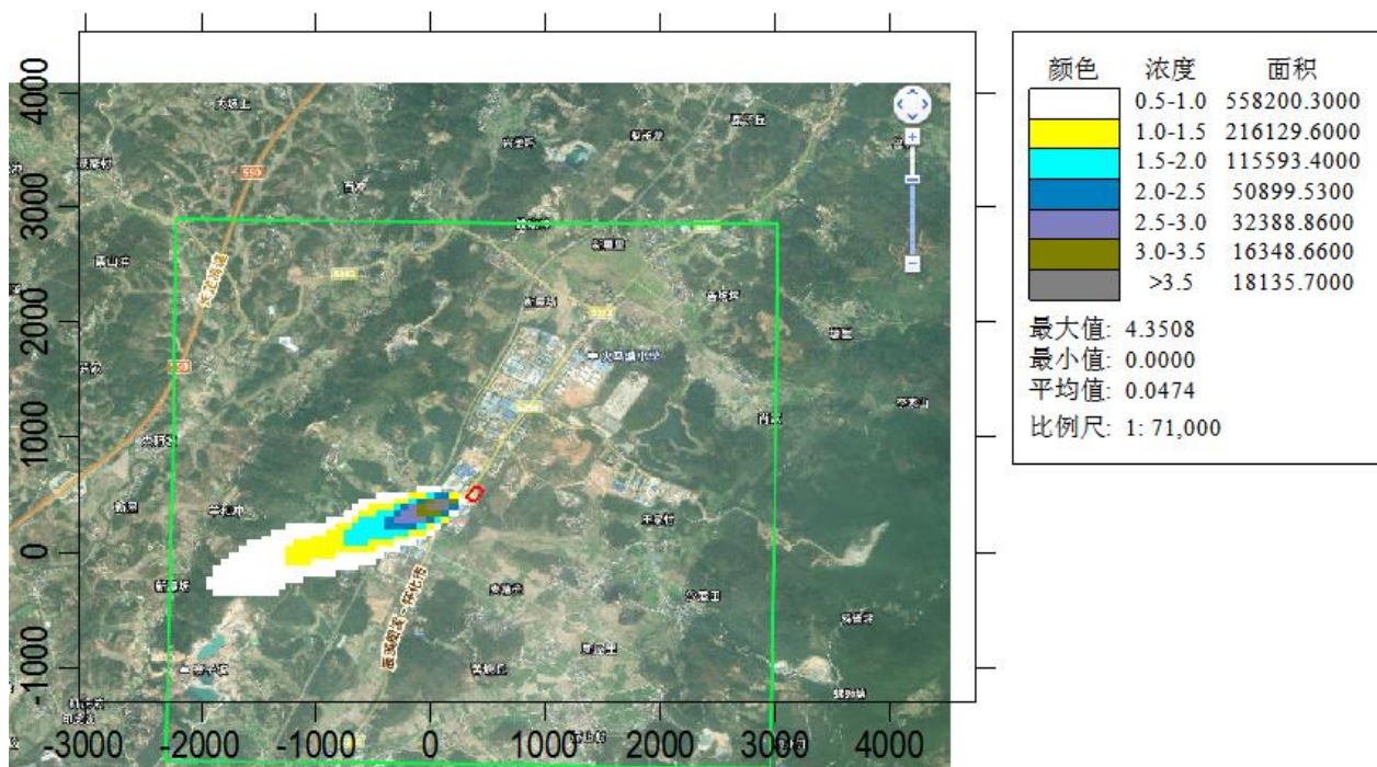
图4.1-10 NO 2 最大小时平均浓度分布图（单位: ug/m 3 ）
