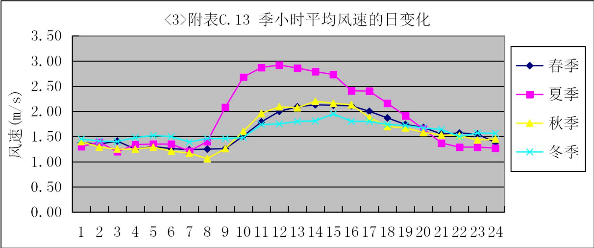
图 4.1-4 怀化市 2024 年季小时平均风速的日变化图
