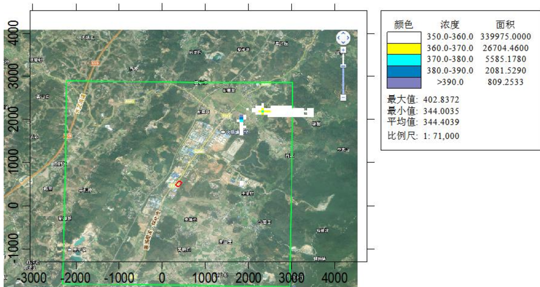
图4.1-26 叠加后TVOC8小时平均浓度分布图（单位： \mu\text{g}/\text{m}^3 ）
