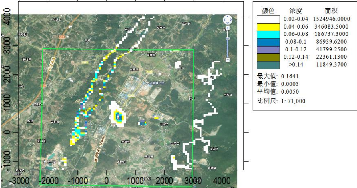
图 4.1-13 PM 10 最大日均值浓度分布图 (单位: ug/m 3 )
