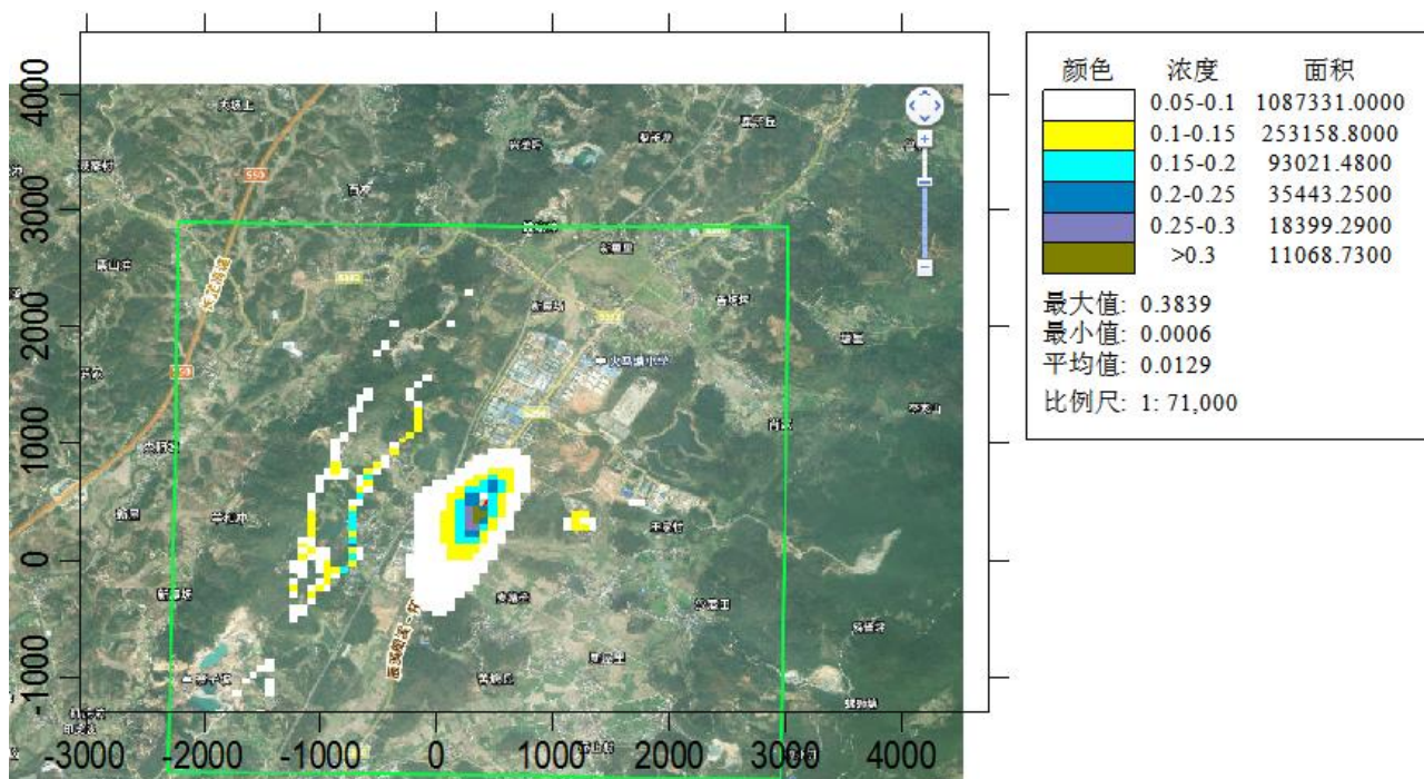
图4.1-12 NO 2 最大年平均浓度分布图（单位：ug/m 3 ）
